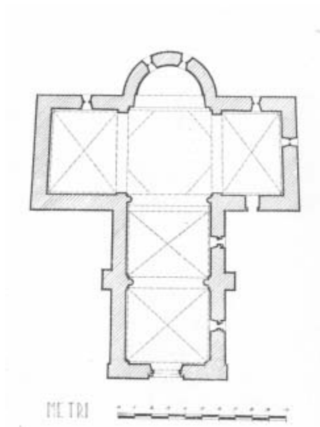
Fig. 183. - Montorfano - S. Giovanni - Pianta
