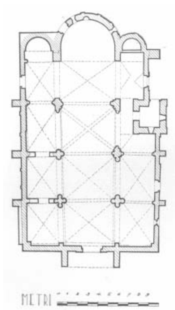
Fig. 226. - Casalvolone - S. Pietro - Pianta
