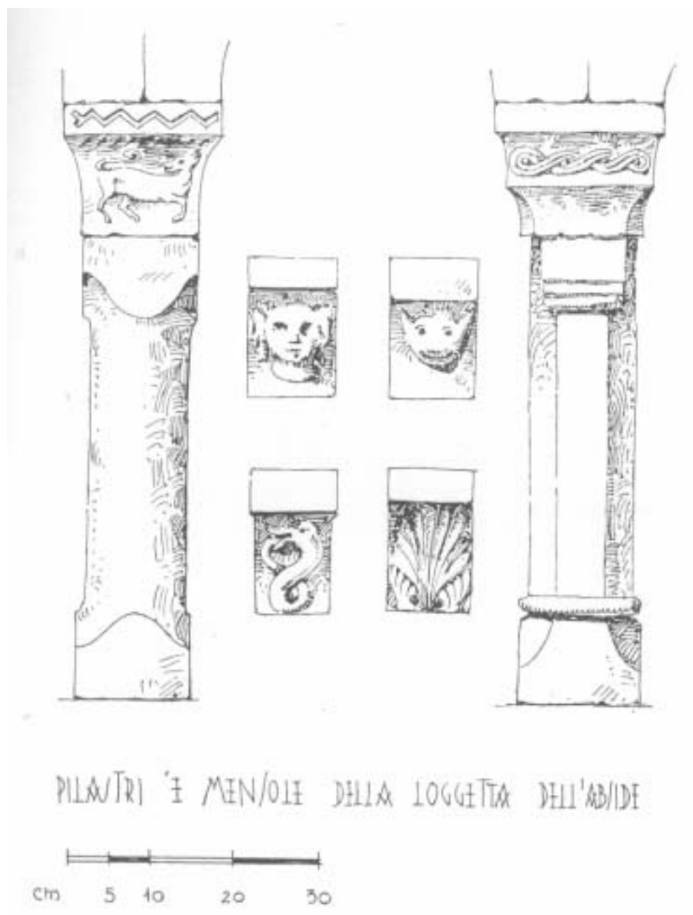
Fig. 191 - Montorfano - S. Giovanni - Particolari
