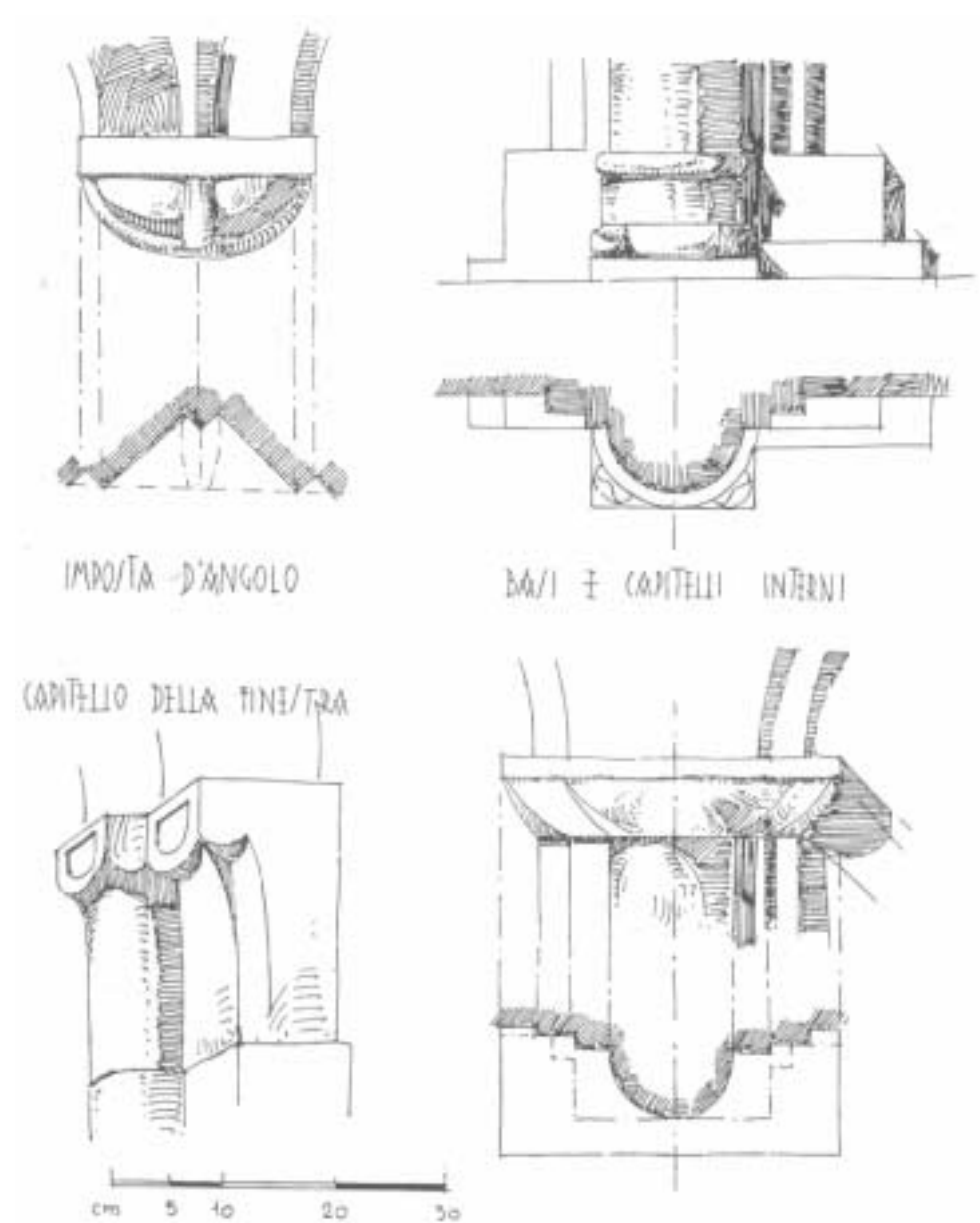
Fig. 188. - Montorfano - S. Giovanni - Particolari
