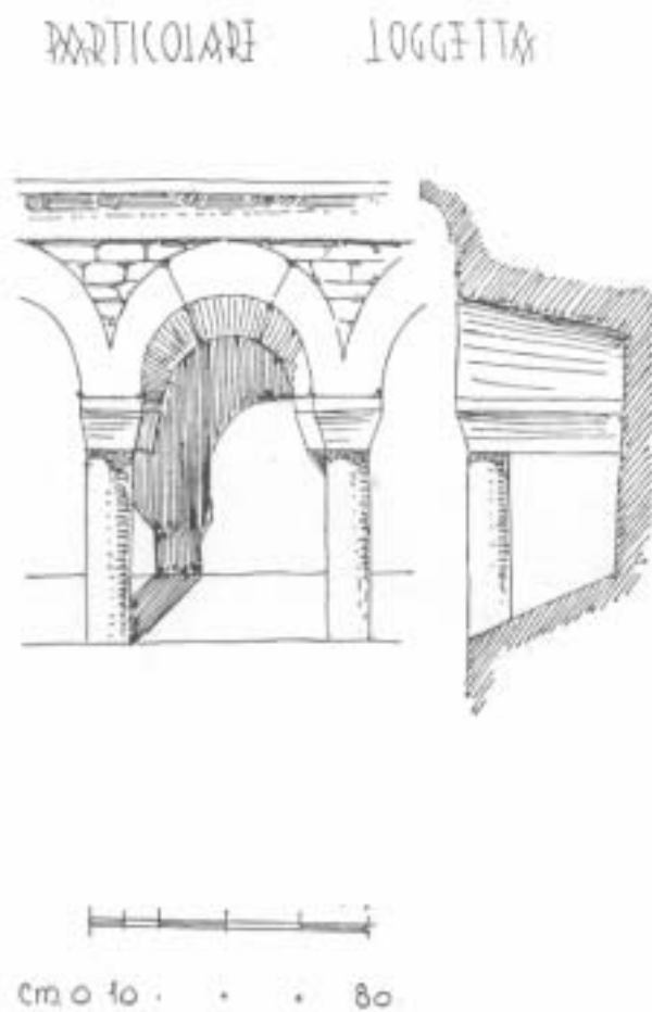
Fig. 192. - Montoffano - S. Giovanni Loggetta dell'abside
