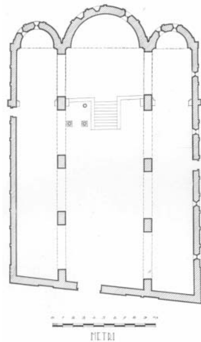
Fig. 216. - Oleggio - S. Michele - Pianta
