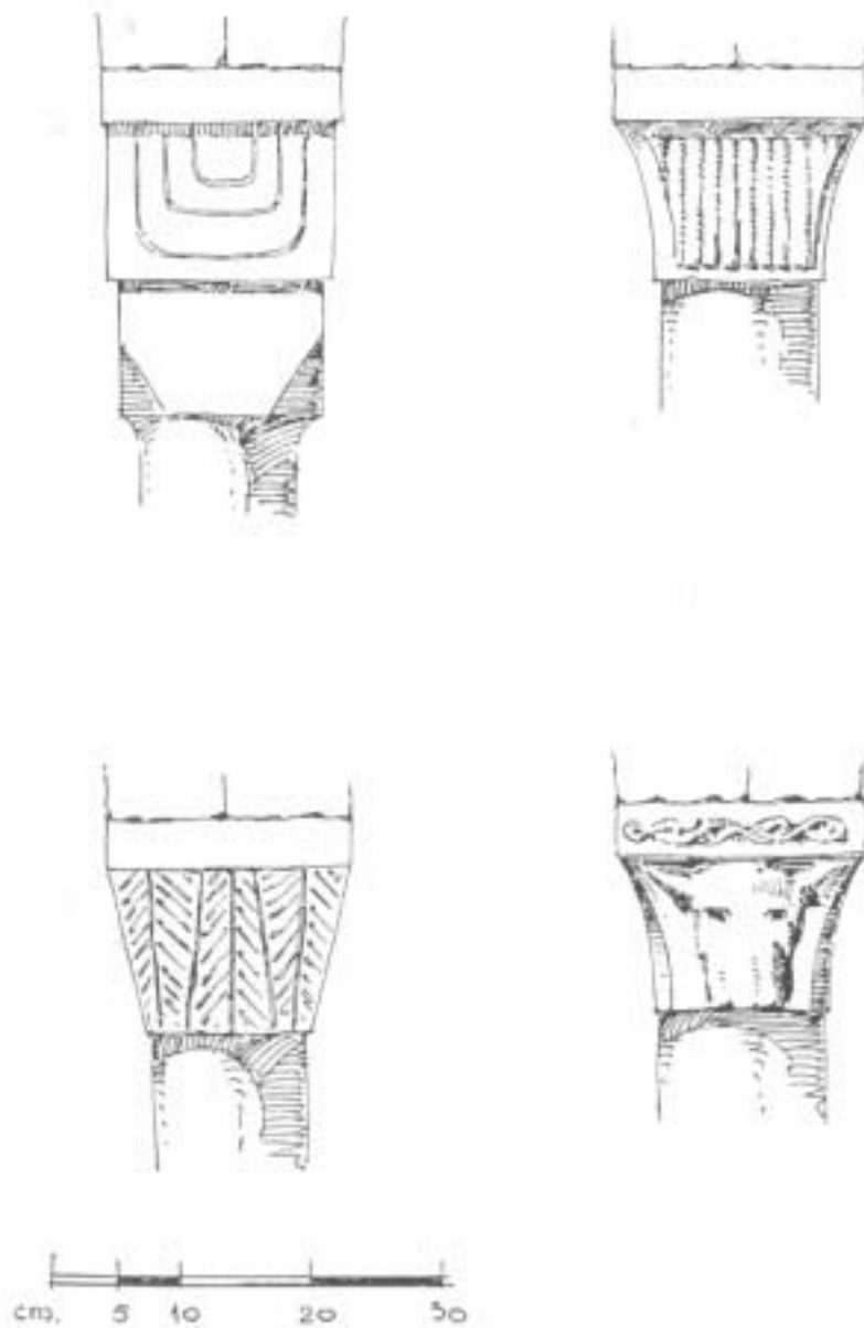
Fig. 190. - Montorfano - S. Giovanni - Particolari
