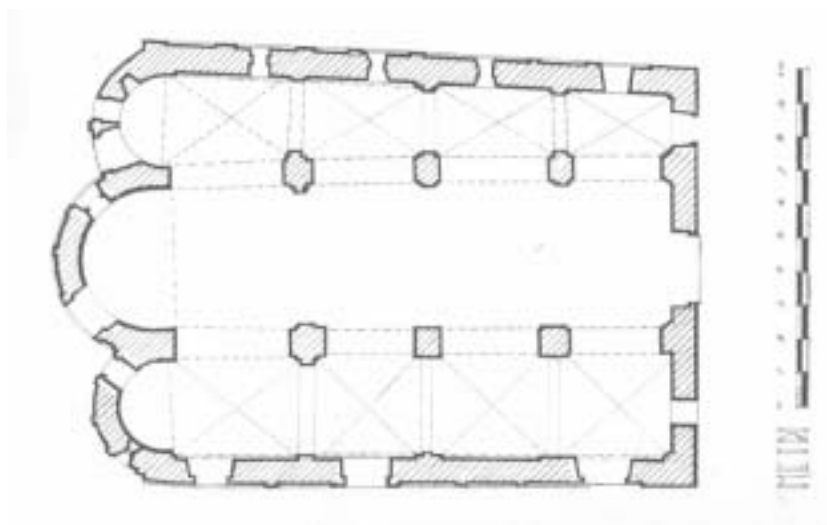
Fig. 211. - Carpignano - S. Pietro Pianta
