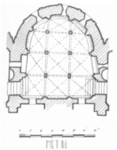
Fig. 217. - Oleggio S. Michele - Cripta
