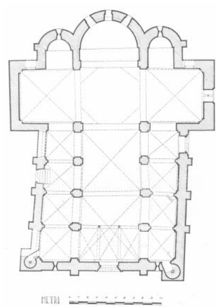
Fig. 238. - Orta S. Giulio - Pianta 1/200
