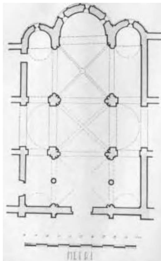
Fig. 172. - Dulzago - S. Giulio - Pianta
