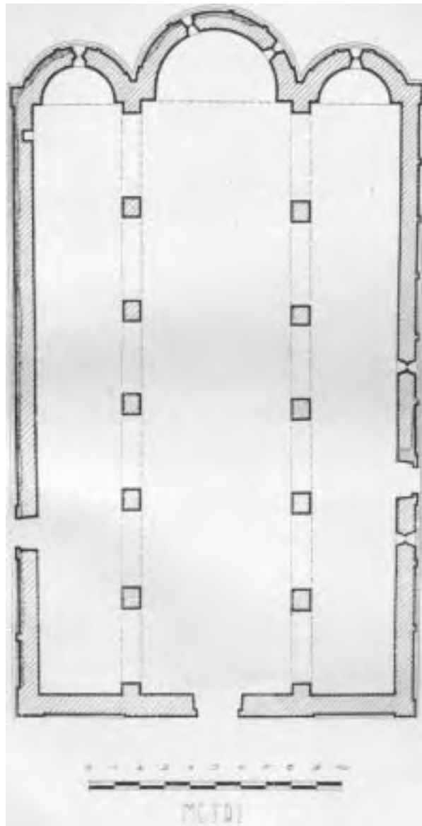
Fig« 132 - Cattico - S. Martino - Pianta
