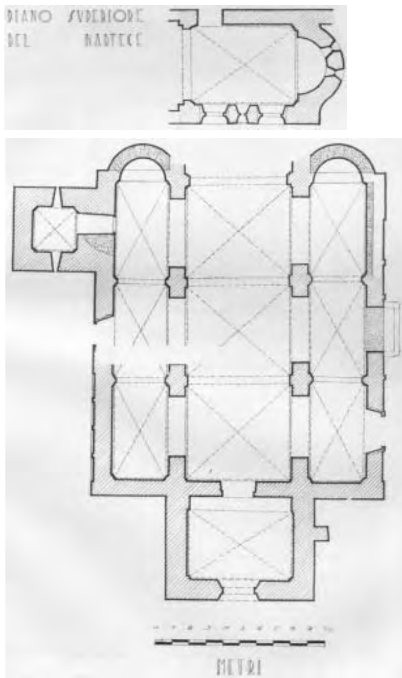
Fig. 167. - Pombia - S. Vincenzo - Pianta
