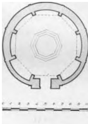
Fig. 140. - Agrade Conturbia - Battistero Pianta
