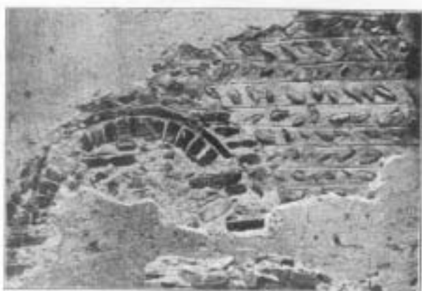
Fig. 52. - Cavaglietto - S. Pietro Particolare del muro a giorno
