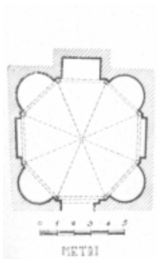
Fig. 22. - Baveno - Battistero Pianta
