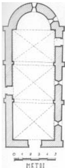
Fig. 24. Borgomanero - S. Leonardo Pianta originale
