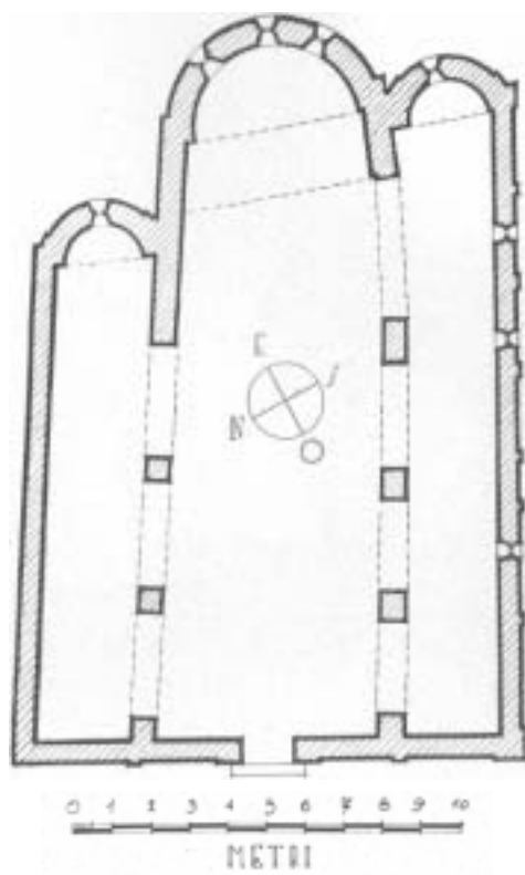
Fig. 12. - Casalino - S. Pietro Pianta originale
