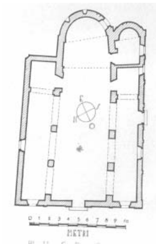
Fig. 11. - Casalino - S. Pietro Pianta allo stato attuale
